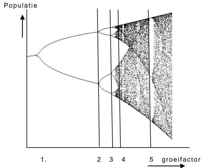
Fig. 10. Bifurcaties (tweesplitsingen) in de oplossing van de logistische vergelijking voor het populatieniveau bij beperkte voedselvoorziening. Let op de witte banden met orde in het chaotische gebied.
