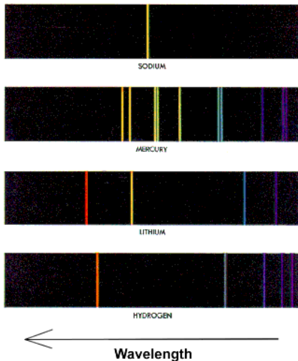
Fig. 3. Spectra van bekende atomen.
