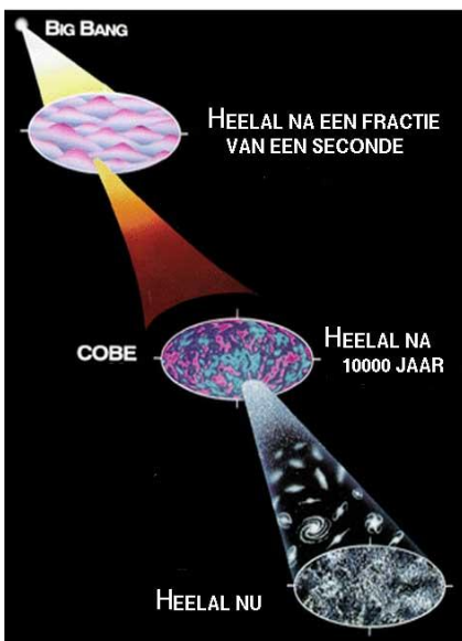
Fig. 4. De ontwikkeling van het heelal na de Oerknal.
