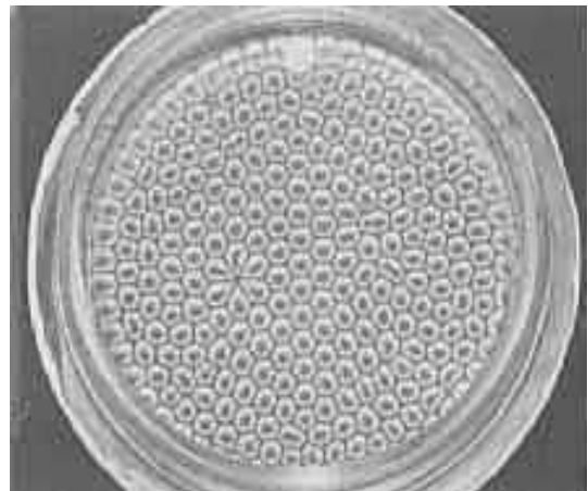
Fig. 8. Bovenaanzicht van de Bénardcel [10]
